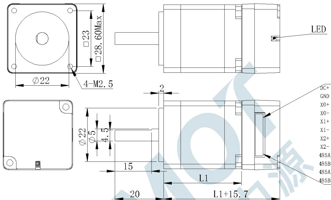
图 1 安装尺寸图 (单位: mm)
