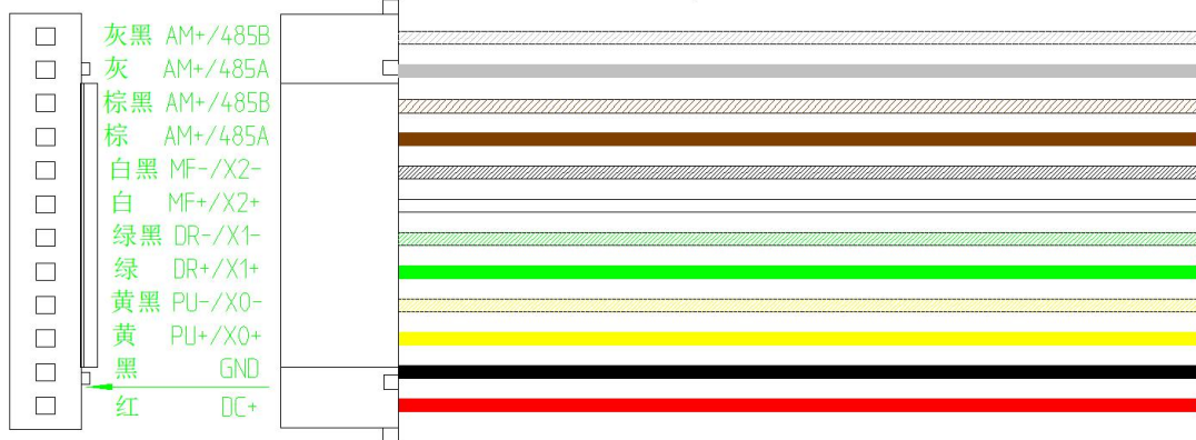
图 6.2 IRS28(E)系列配线示意图
