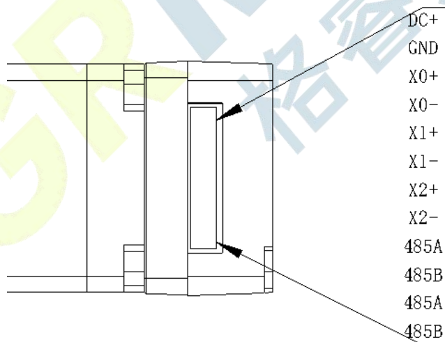
图 3.2 IRS28(E)一体式 485 总线型开(闭)环步进驱动器接口示意图
