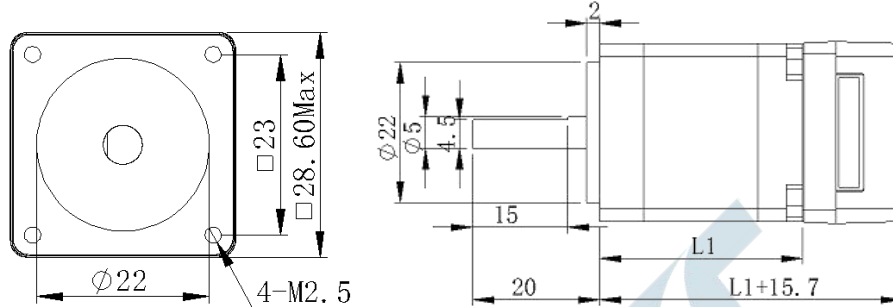
图 6.1 IRS28(E)系列一体机外观示意图
