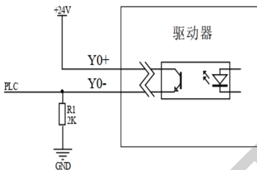
图 3.6 输出接口常闭接法示意图
