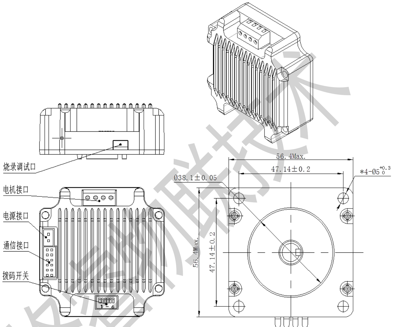
图 1 安装尺寸图 (单位: mm)
