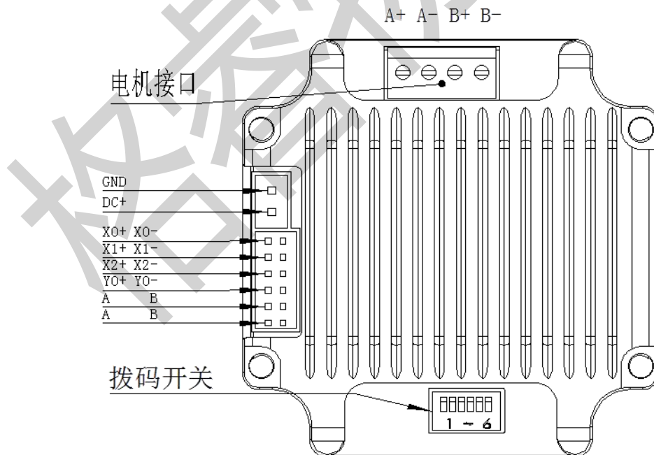
图 3.1 IRS57E 接口示意图
