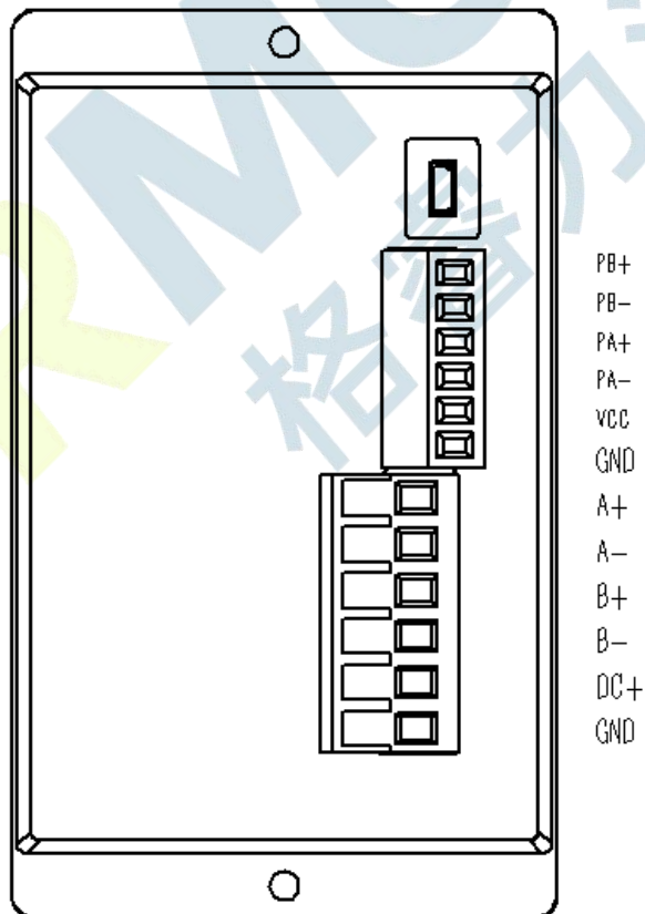
图 3.1 SCT1-86E 接口示意图
