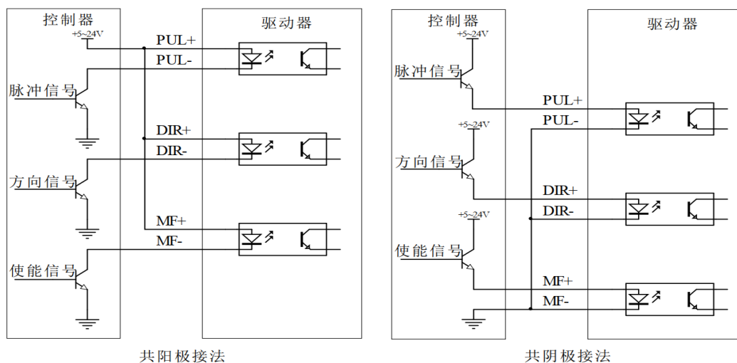
图 2 输入接口电路
