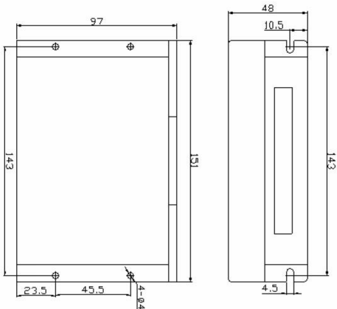
正面安装图
